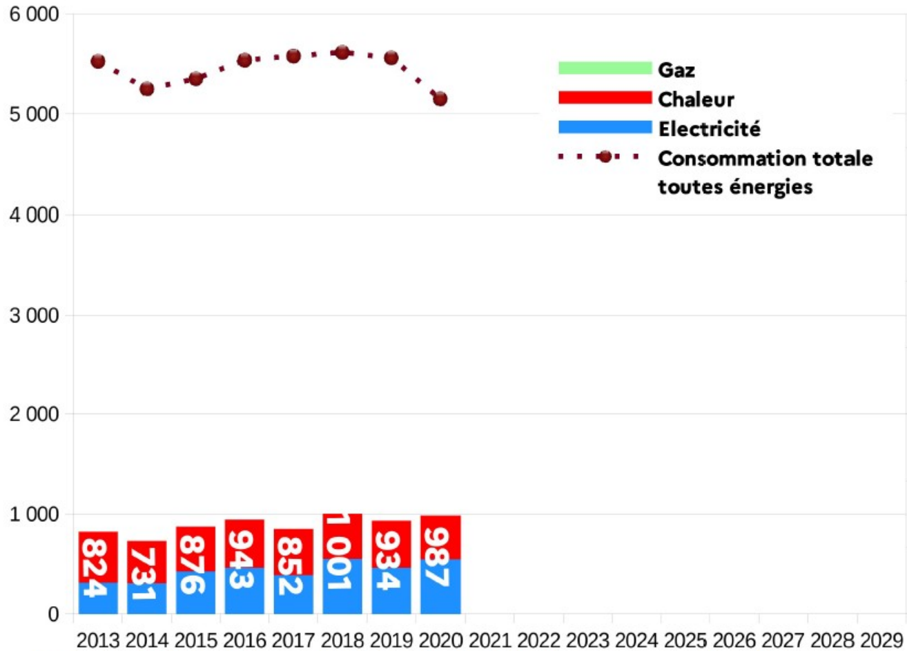
Fig.3 : évolution de la production d'EnR et de la consommation d'énergie du Tarn-et-Garonne (GWh)
